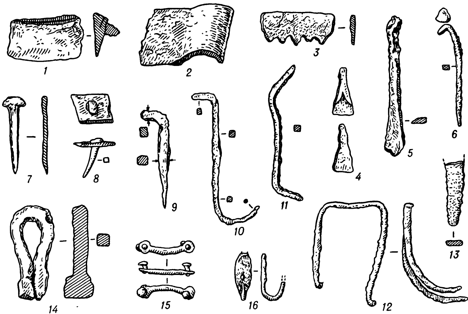
Каменское городище. Изделия из железа: 1 — лезвие топора; 2 — обух топора; 3 — обломок пилы; 4 — долотце; 5 — перка; 6 — гвоздь с боковой шляпкой; 7 — гвоздь из пластины; 8 — обойный гвоздь; 9 — костыль; 10 — крюк стеной; 11 — соединительная скоба; 12 — скоба для укладки орудий; 13 — ножевидный стеной шип; 14 — дверная петля; 15 — скрепка с клепками; 16 — овальная скрепка с шипами.
